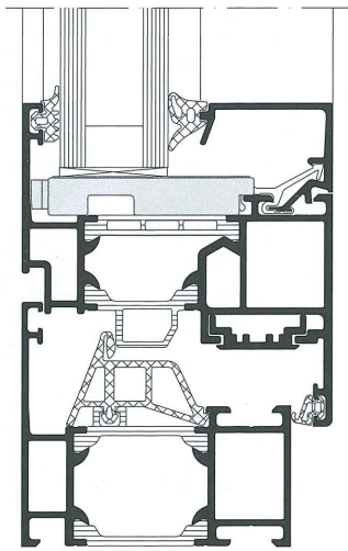
AWS 65, 比例1:2 AWS 65, Scale 1:2
